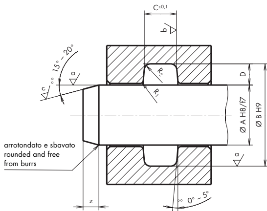
Tenuta per asta, sede nella parete del cilindro Rod packing, groove in cylinder wall
