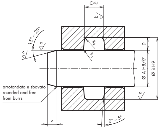
Tenuta stelo, sede nella parete del cilindro Rod packing, groove in cylinder wall
