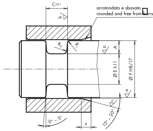
Tenuta per cilindro, sede nel pistone o nell'asta Cylinder packing, groove in piston or shaft
