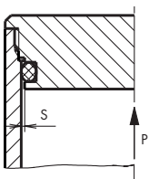
La pressione elevata aumenta l'interstizio di tenuta (errato) High pressure increases sealing gap (wrong)
